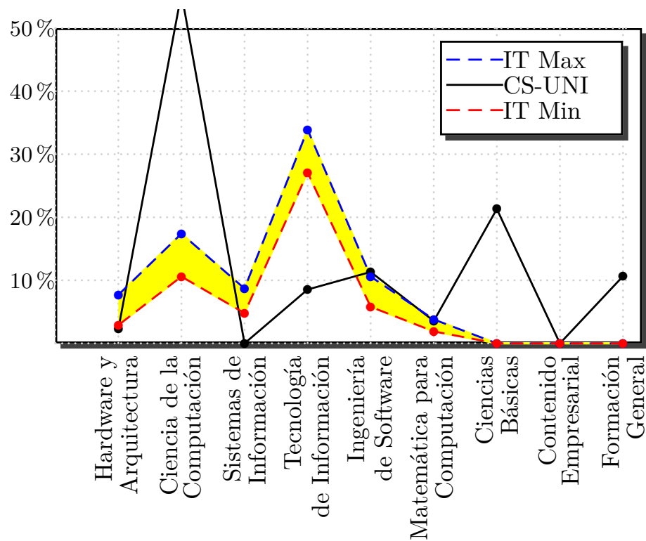
Figura 3.11: Comparación de CS-UNI con IT de ACM/IEEE-CS.
