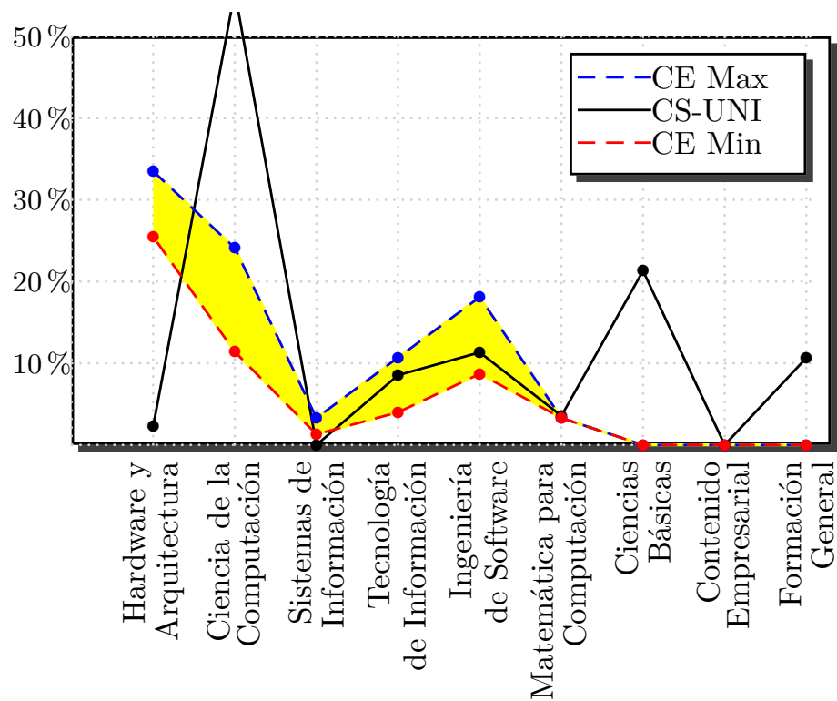
Figura 3.7: Comparación de CS-UNI con CE de ACM/IEEE-CS.
