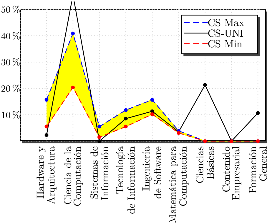
Figura 3.5: Comparación de CS-UNI con CS de ACM/IEEE-CS.
