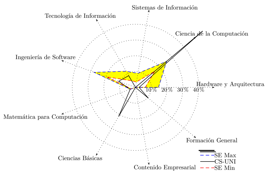
Figura 3.14: Comparación de CS-UNI con SE de ACM/IEEE-CS.
