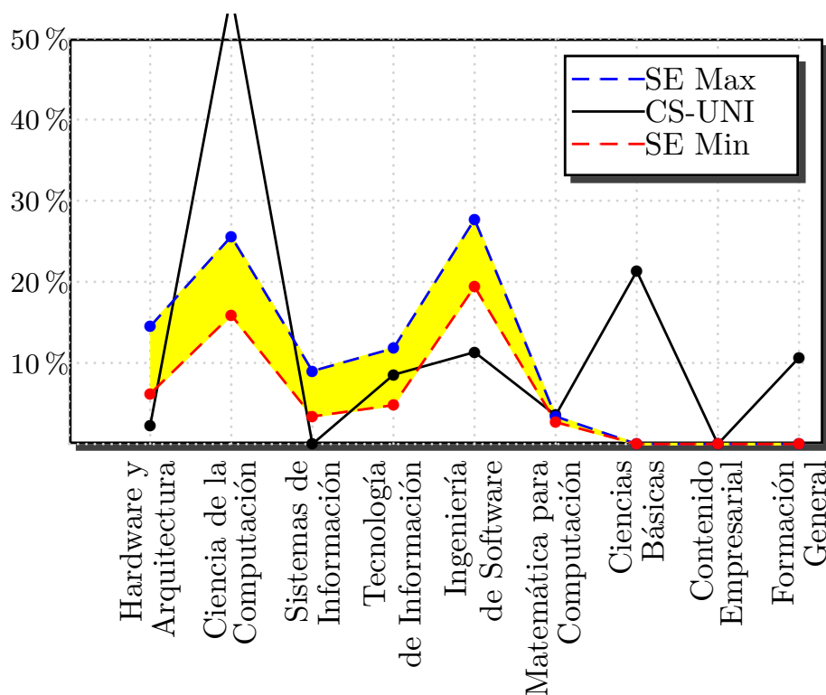
Figura 3.13: Comparación de CS-UNI con SE de ACM/IEEE-CS.
